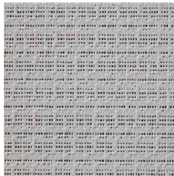
Polyestergewebe Gewebe aus hochfesten Polyesterarnen, in beide Richtungen vorgereckt und PVC-fixiert (Precontraint-Verfahren)
