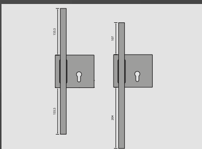
Griffstangen für Schiebetürschloss Pari 2.0: G 420 rund oder G420 eckig/breit
